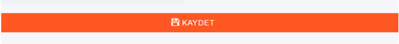
Resim 13:Kaydet butonu
